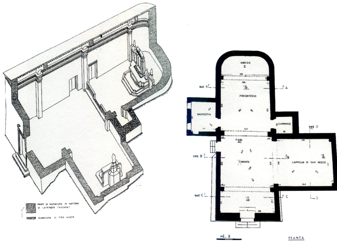
Assonometria e pianta. Campagna di rilievi 1993-1994.
