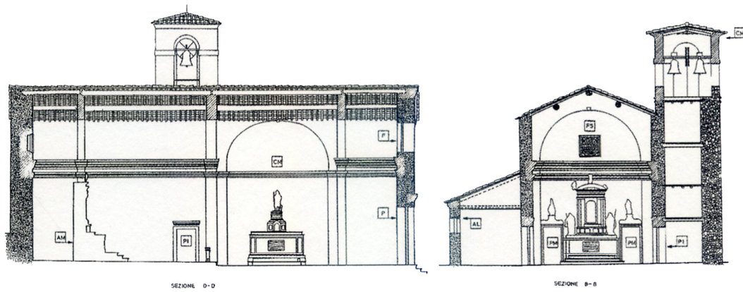
Sezioni longitudinale e trasversale.
