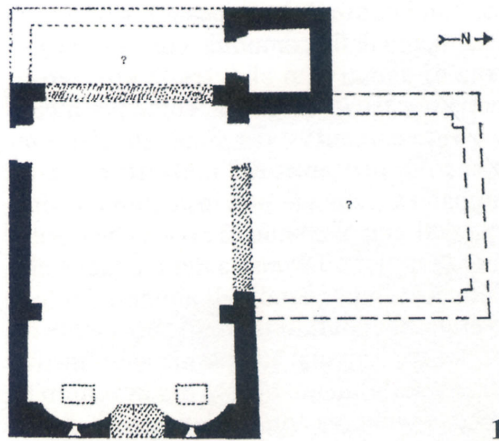
1- Ricostruzione in base ai rilievi architettonici del 1994 e al verbale della visita vescovile del 12 ottobre 1488.
