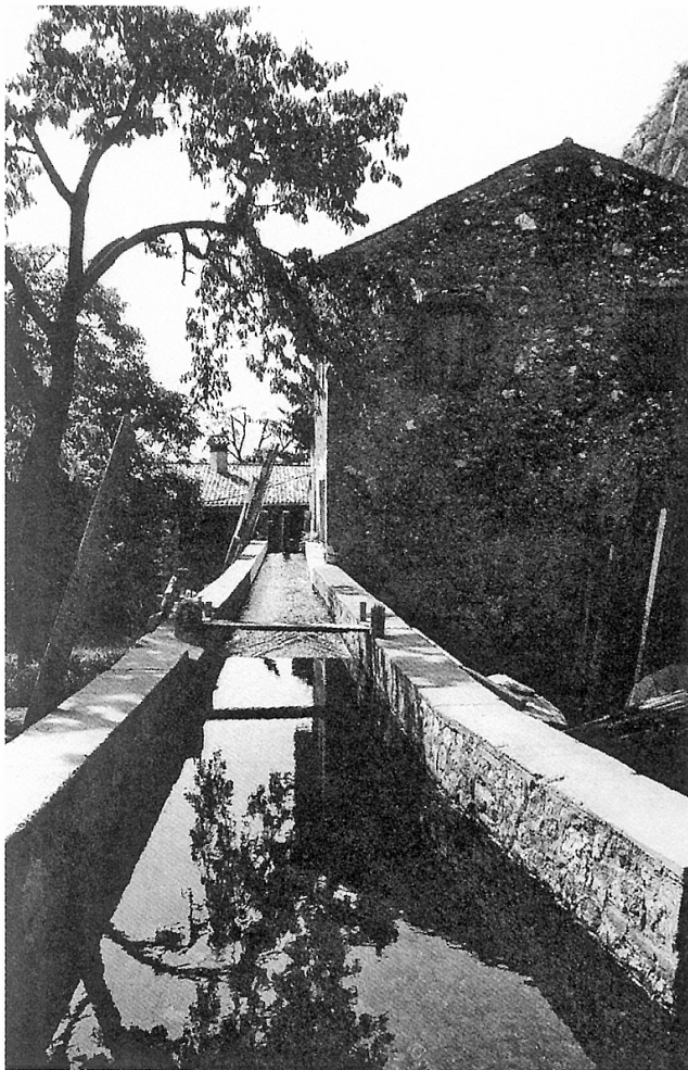
Casa del munaro; parte finale del canale di derivazione tra la presa dell'acquedotto del Monastero (a sinistra) e il salto con il partitore per le due ruote idrauliche.
